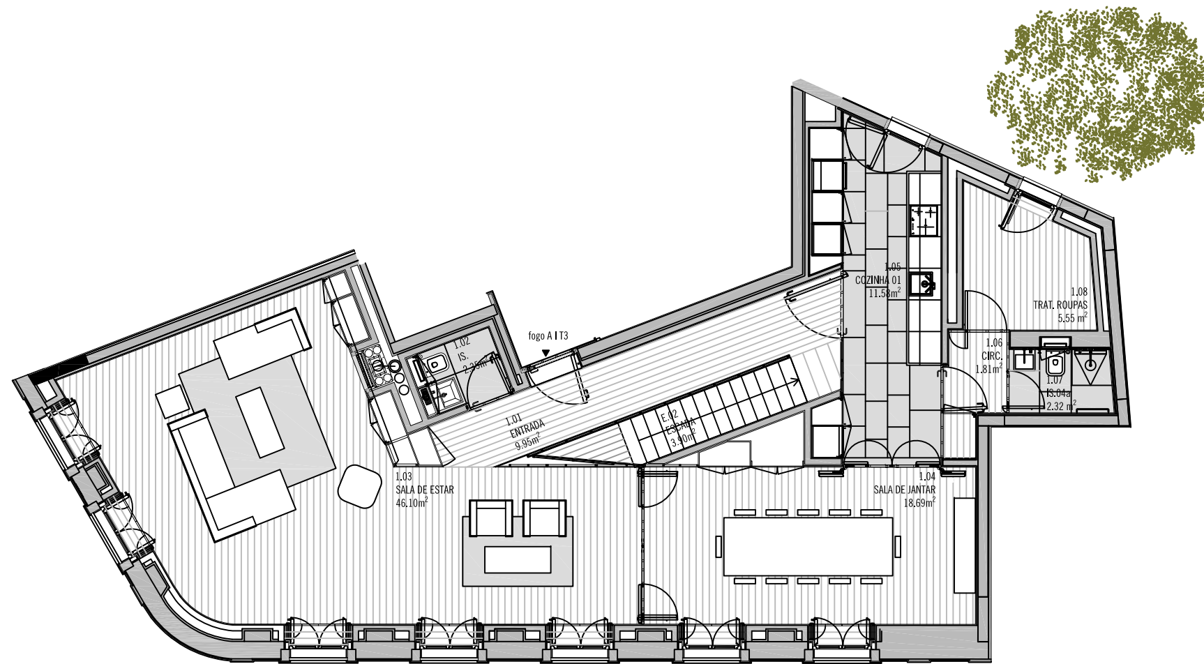
PISO 1
